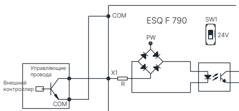
Рис. 3-14 Подключение встроенного источника питания 24 В в режиме «Источник»
