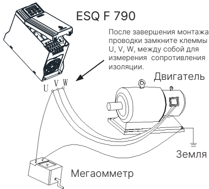
Рис. 1-1 Проверка изоляции мотора
