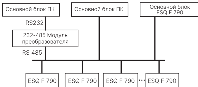
Рис. В-1 Схематическая диаграмма способа организации сети
