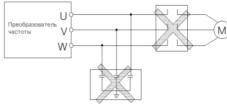
Рис. 3-6 Запрещено использовать контактор и фильтрующий конденсатор
