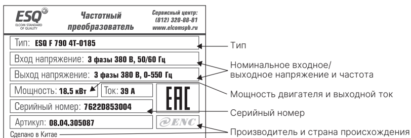
Рис. 2-2 Шильда
