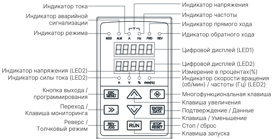
EN-LED16 Схема расположения клавиш Рис. 5-2 Устройство панели управления
