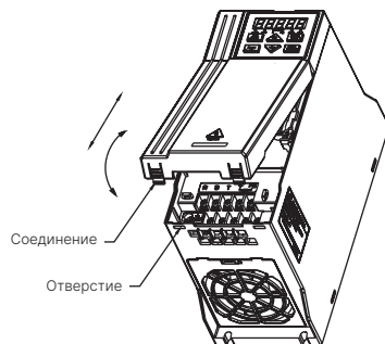
Fig. 3-4 Установка и снятие крышки
