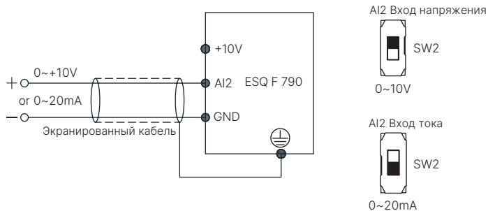
Рис. 3-12 Схема подключения клеммы AI2
