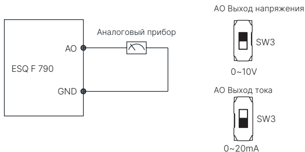
Рис. 3-13 Схема подключения клемм AO
