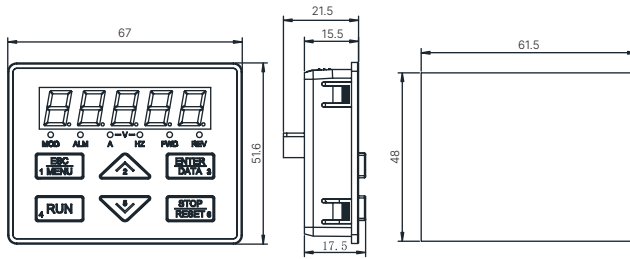
Рис. 2-5 EN-LED15 внешний вид и размеры отверстия клавиатуры
